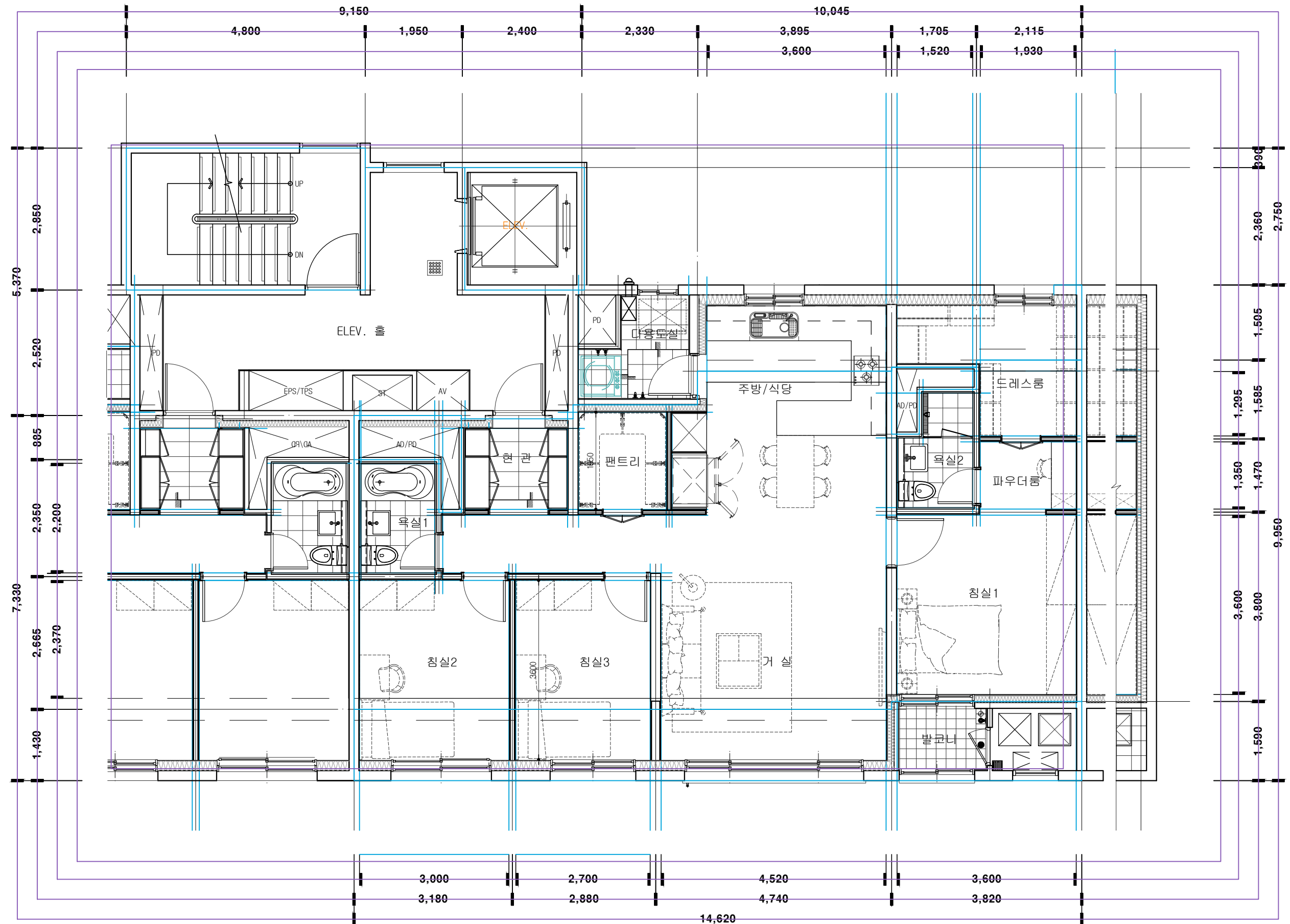
84A-단위세대평면도 SCALE : 1 / 80
